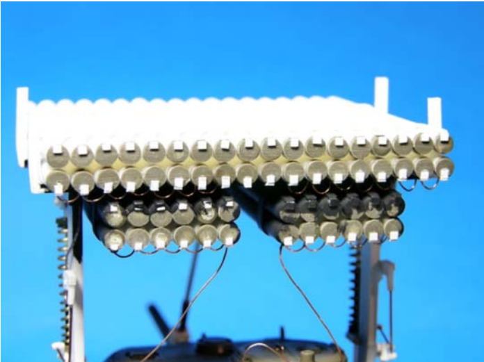
Vista posteriore del sistema lanciarazzi T34 realizzato con tubolari Evergreen di diametro adeguato
