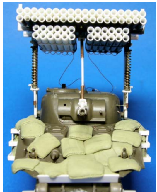
Vista della parte frontale dello scafo, ricoperta anch'essa con sacchetti di sabbia riprodotti in Milliput
