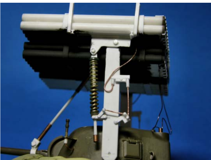
Dettaglio laterale dell'impianto per il sostegno e l'alzo del sistema d'arma, azionato tramite il braccio collegato al cannone da 75 mm.
